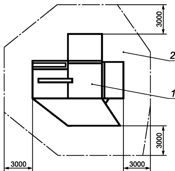
1 — фанбокс; 2 — зона безопасности
