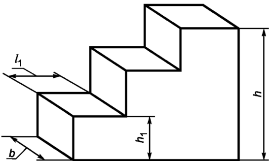
Рисунок 14 — Лестница
