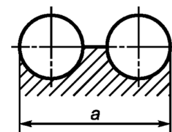
Рисунок 3 — Параллельное расположение ребер
