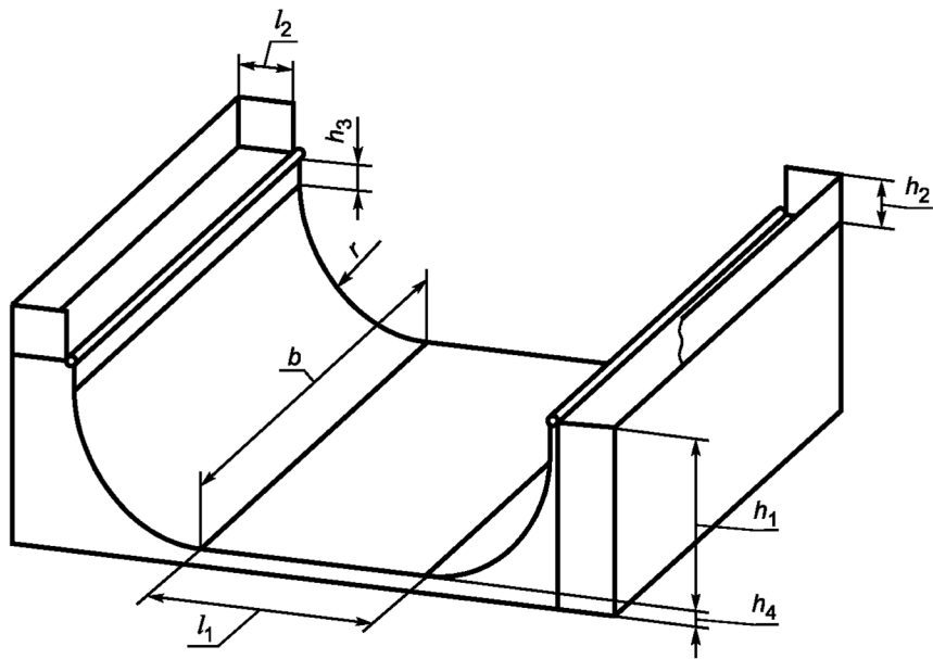
Рисунок 15 — Пайп
