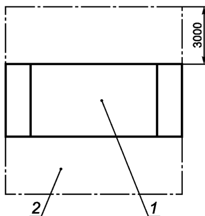
1 — мини-пайп; 2 — зона безопасности
