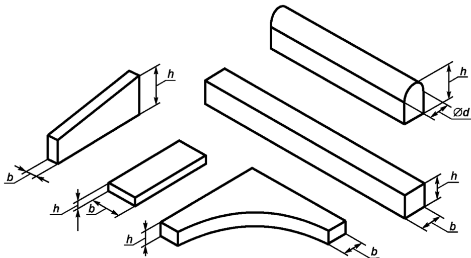
Рисунок 6 — Уступ
