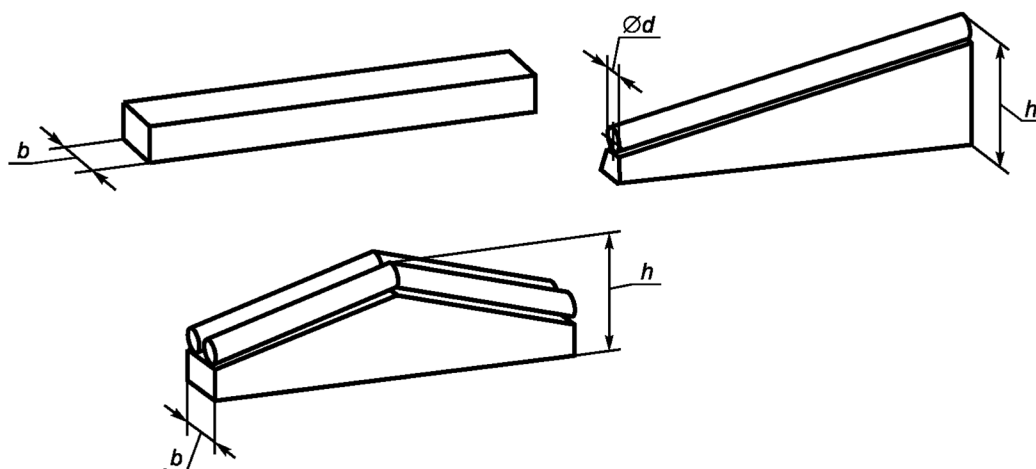
Рисунок 5 — Бордюры
